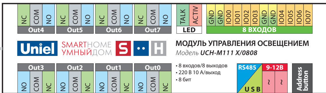
ВЫХОДЫ УПРАВЛЯЮЩИХ РЕЛЕ ДЛЯ ПОДКЛЮЧЕНИЯ ИСТОЧНИКОВ СВЕТА
